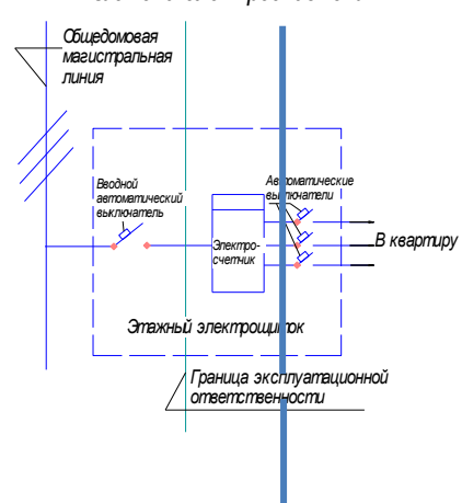
Рис. 4 Система электроснабжения
