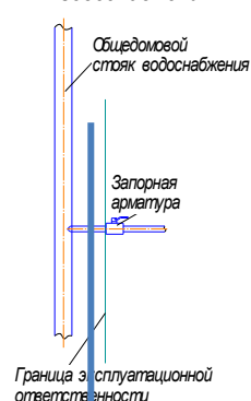
Рис. 2 Система холодного и горячего водоснабжения
