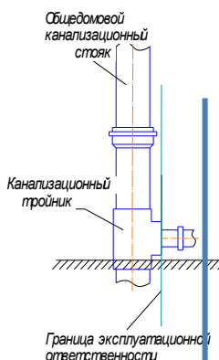
Рис. 3 Система водоотведения
