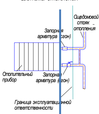
Рис. 1 Система отопления
